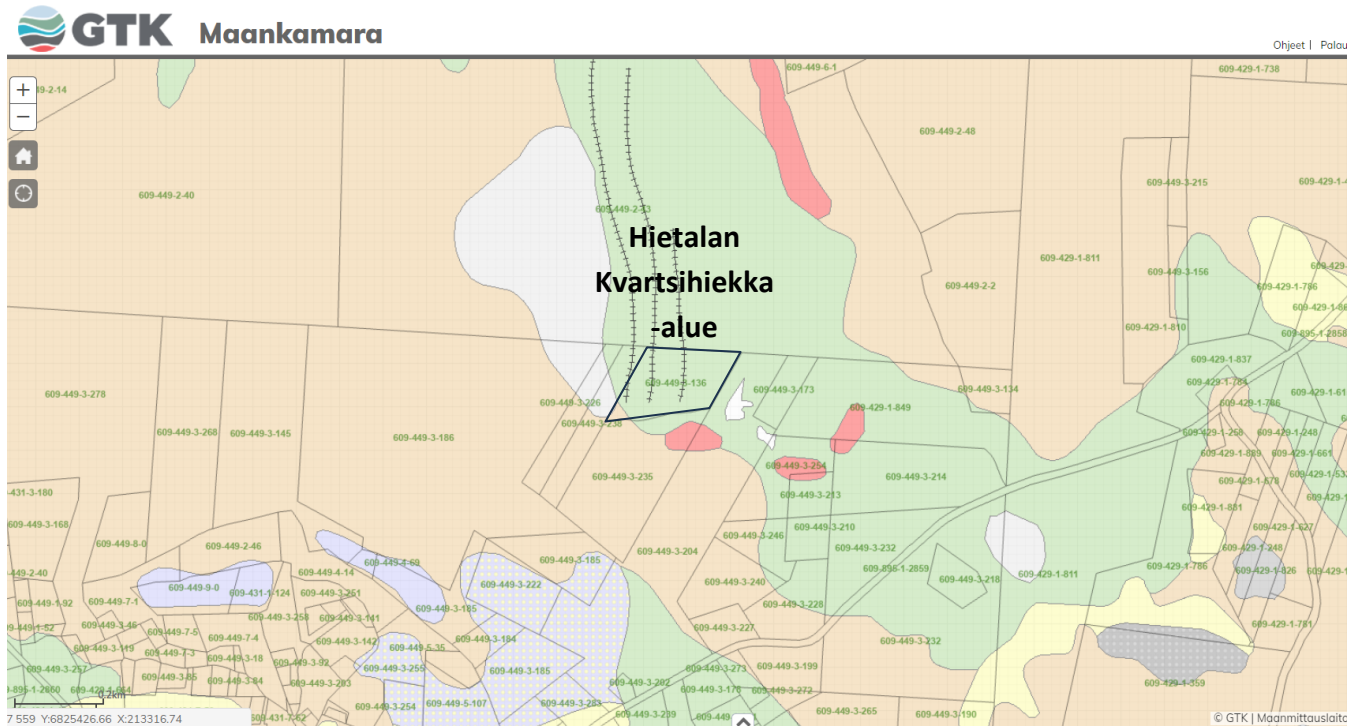
Kuva 1. Maaperäkarta. Hietalan tila on osoitettu rajauksella. Ottamisalueen tilan alueella on jäätikkökijokimuodostuma, joka on hiekkaa. Ottamisalueella tehtyjen havaintojen mukaan esiintymä on kvartsiptoista hiekkaa. Mittajana 0,2 km on kartan vasemmassa alakulmassa. Lähde: GTK, Maanmittauslaitos, Esri Finland.
