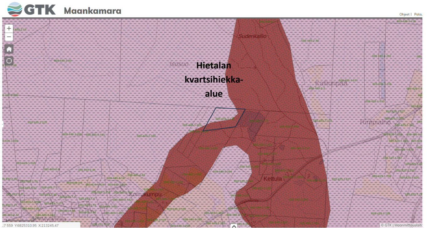
Kuva 2. Kallioperäkarta. Hietalan tila on osoitettu rajauksella. Ottamisalueen kallioperä, irtaimien maa-ainesten alla, koostuu kahdesta kiviaineslajista eli Jotuninen Satakunnan hiekkakivi (läntinen osa-alue) ja Postijunainen oliviinidiabaasi (itäinen osa-alue). Mittajana 0,2 km on kartan vasemmassa alakulmassa. Lähde: GTK, Maanmittauslaitos, Esri Finland.
